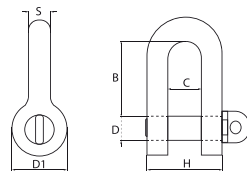
PERNO OLHAL
