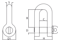
PERNO OLHAL
