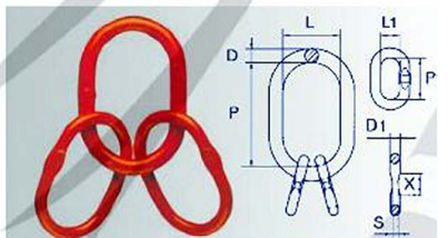
Argo ão oval conjunto para lingas de 3 ou 4 ramais Special sub-assembly
