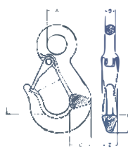
Gancho de olhal com patilha de segurança Din.7541 Lifting eye hook DIN 7541 degree 8
