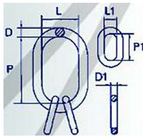
Argolão oval conjunto para lingua de 3 ou 4 ramos Sub-assembly
