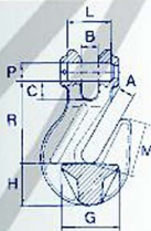
Gancho de forqueta com e sem segurança Fork hook with/without latch
