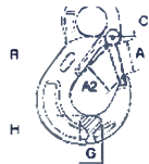
Gancho de olho com patilha de segurança Sling hook with latch
