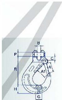
Gancho de forqueta com patilha de segurança Clevis sling hook with latch
