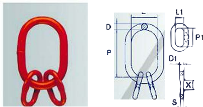
Argolão oval conjunto para lingas de 3 ou 4 ramais Sub-assembly
