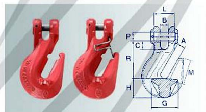
Gancho de forqueta com e sem segurança Fork hook with/without latch
