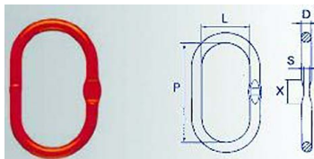
Argolão oval simples para lingas de 1 ou 2 ramais Oblong masterlink
