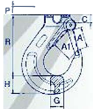
Gancho de forqueta com patilha de segurança Clevis sling hook with latch
