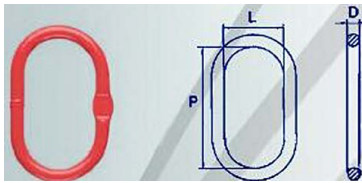
Argolão oval simples para linguas de 1 ou 2 ramos Oblong masterlink
